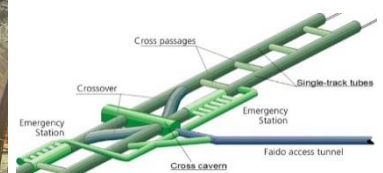
Schema der geplanten Anlage Faido MF
